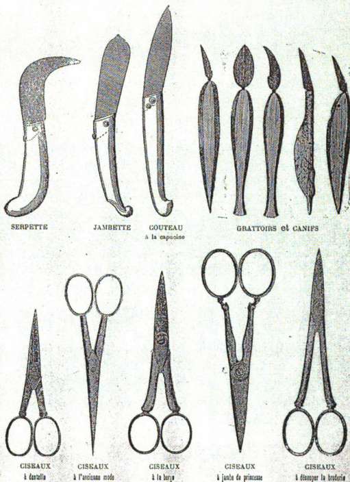
Figure A-41: Knives and scissors in Pagé's La Coutellerie Depuis L'origin Jusqu'a Nos Jours , 1896 Tome I, Partie 1&2, Page 36 bis, Planche XI. Note the Jambette.
